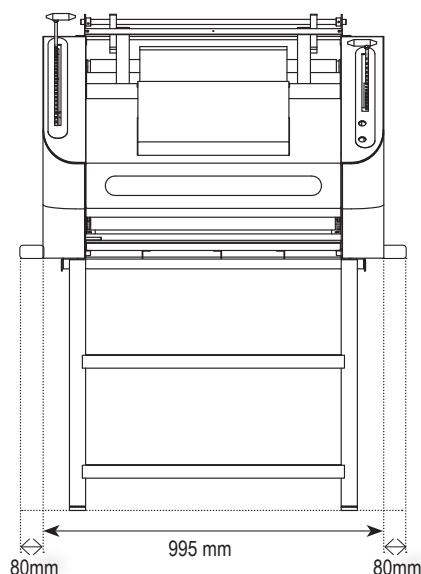
VUE DE FACE ■ FRONT VIEW ■ VOORAANZICHT
