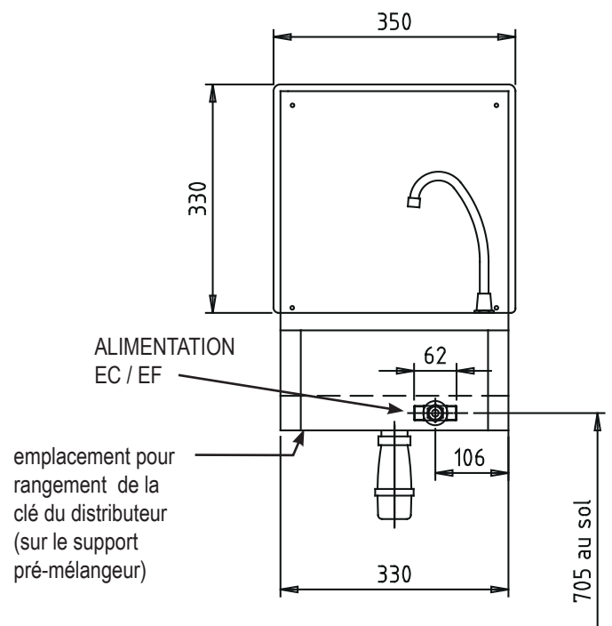
Lave-mains avec dosseret et distributeur de savon, réf. 806 333
