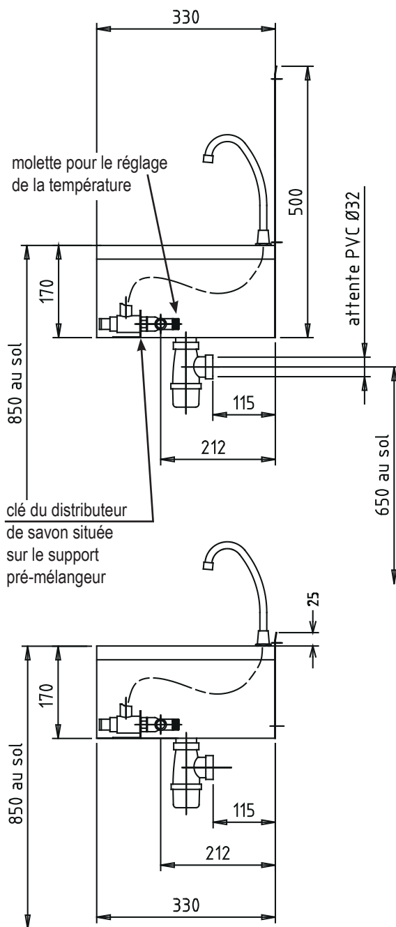
Lave-mains sans dosseret, réf. 806 331
